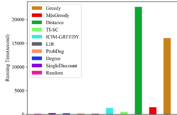
شکل ۱۳- زمان اجرای الگوریتم‌های متفاوت بر روی دیتاست M-FO115
